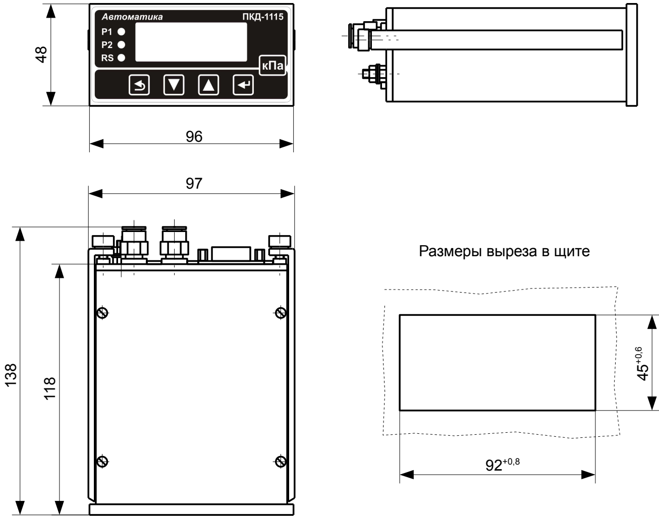
Рисунок А.1 - Габаритные и монтажные размеры прибора щитового исполнения ПВД-1115. ... Щ48
