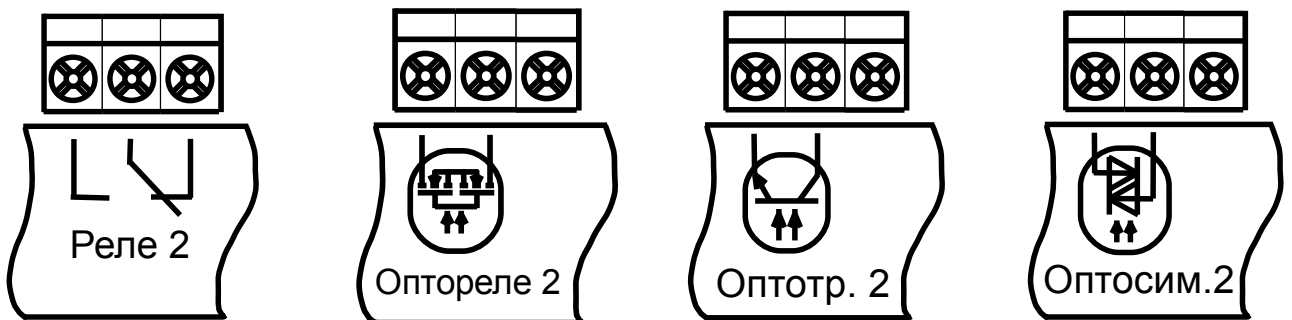
а) электромагнитное реле (сухой контакт)
